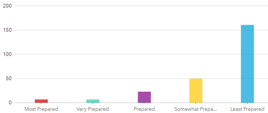
g. Hurricane
